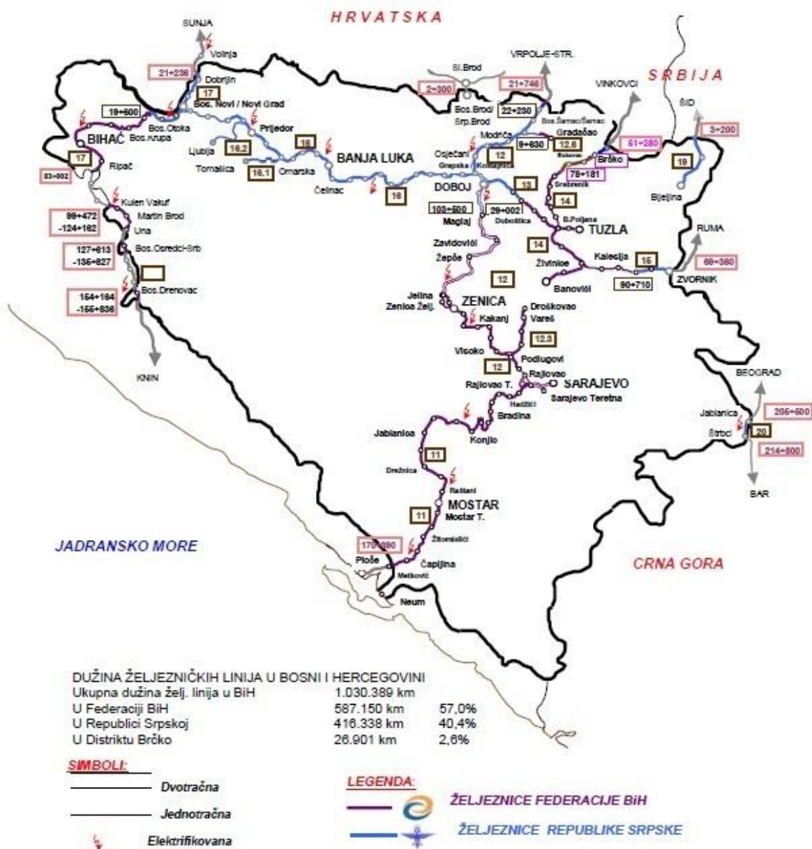
Željeznička mreža Bosne i Hercegovine
